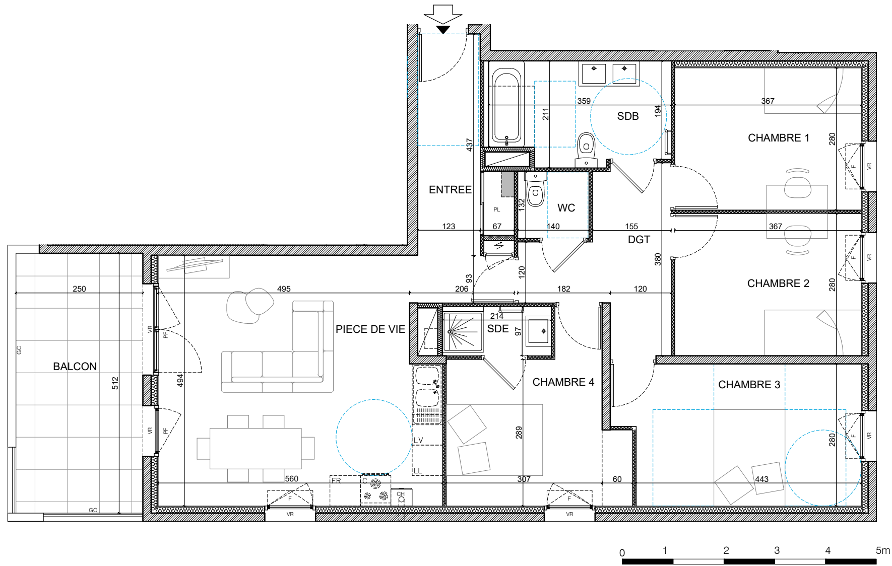
Plan du 1 er étage
